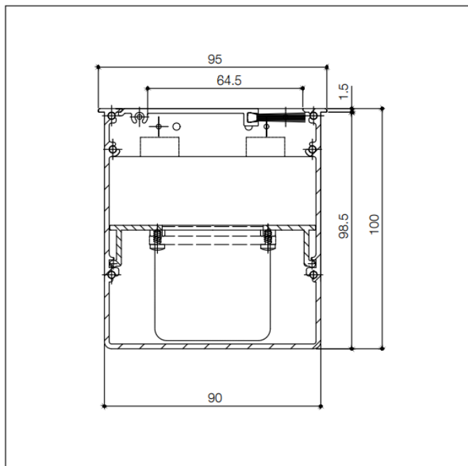
Misure tecniche sezione laterale
