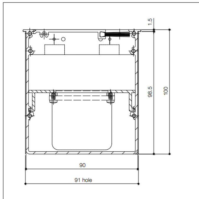
Misure tecniche foro in sezione laterale
